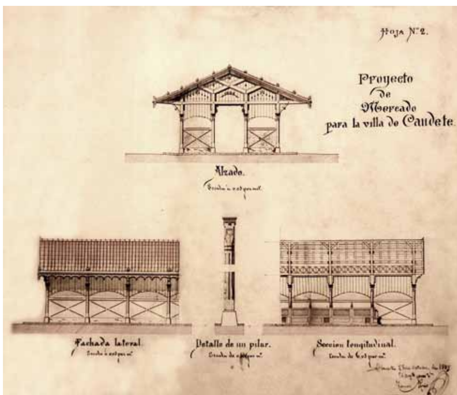
Fig. 2. AMC, Proyecto de obras para la construcción de un Mercado en la Villa de Caudete, C.148, 2. Alzado, fachada lateral, detalle y sección longitudinal.
