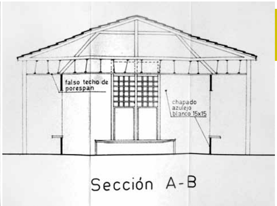
Fig. 7. AMC, Obras de reforma y acondicionamiento del mercado municipal de Caudete. C. 148, 4. Sección transversal.
