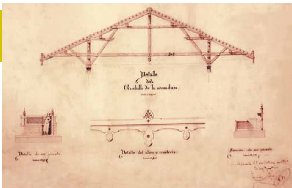
Fig. 3. AMC, Proyecto de obras para la construcción de un Mercado en la Villa de Caudete, C.148, 2. Detalles: estructural, sección y alzado de un puesto, crestería.
