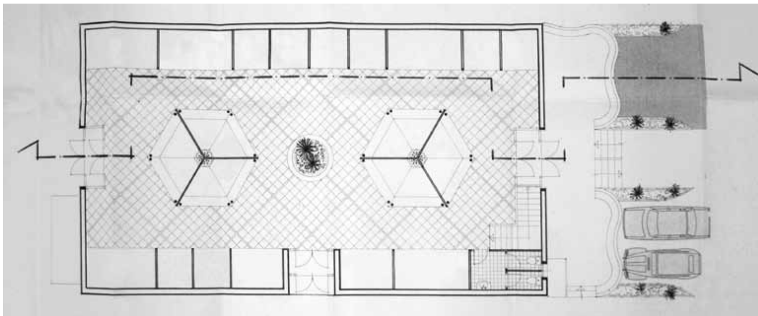
Fig. 8. AMC, Proyecto de rehabilitación del Mercado Municipal. C. 149. Planta baja.
