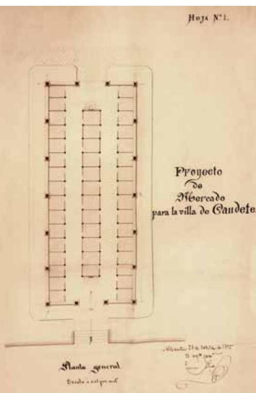
Fig. 1. AMC, Proyecto de obras para la construcción de un Mercado en la Villa de Caudete, C.148, 2. Planta.
