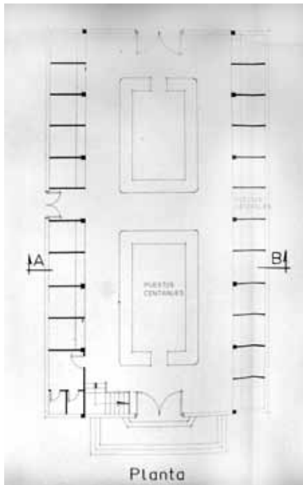
Fig. 6. AMC, Obras de reforma y acondicionamiento del mercado municipal de Caudete. C. 148, 4. Planta.
